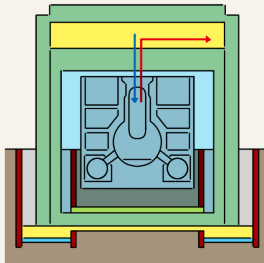
冠水工法の一例
