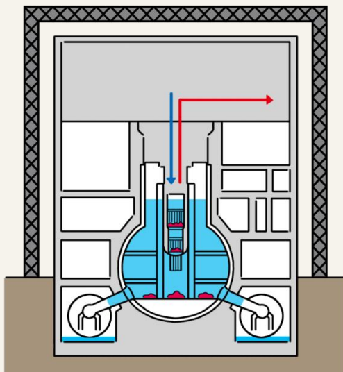
気中工法の一例 (上アクセスと横アクセスの組合せ)
